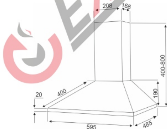
Рис. 1 Внешний вид кухонной вытяжки и схема размеров
